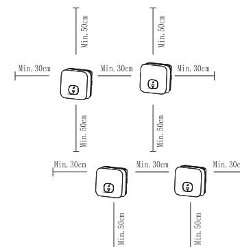
Distanze di rispetto per una serie di inverter
