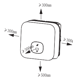
distanze di rispetto per un inverter
